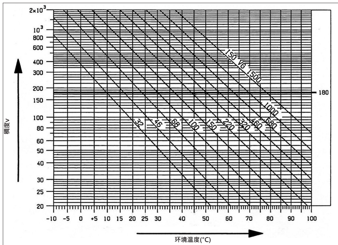
稠度/环境温度图表 mm 2 /s = cSt
